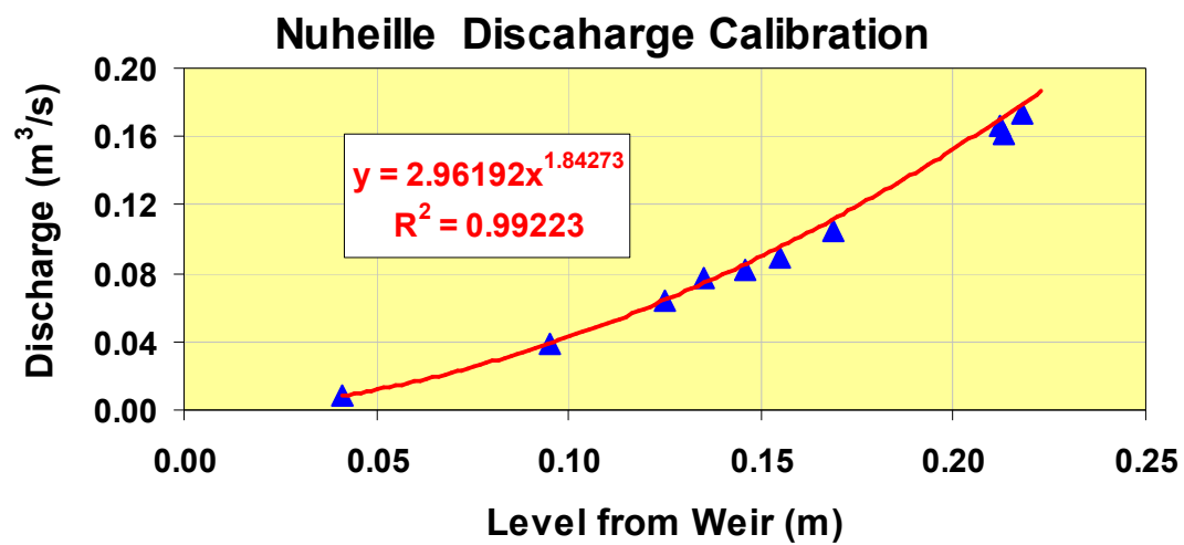
איור 2 : גרף כיול למד המפלס הרציף שהותקן בתעלת הנוחיילה.
